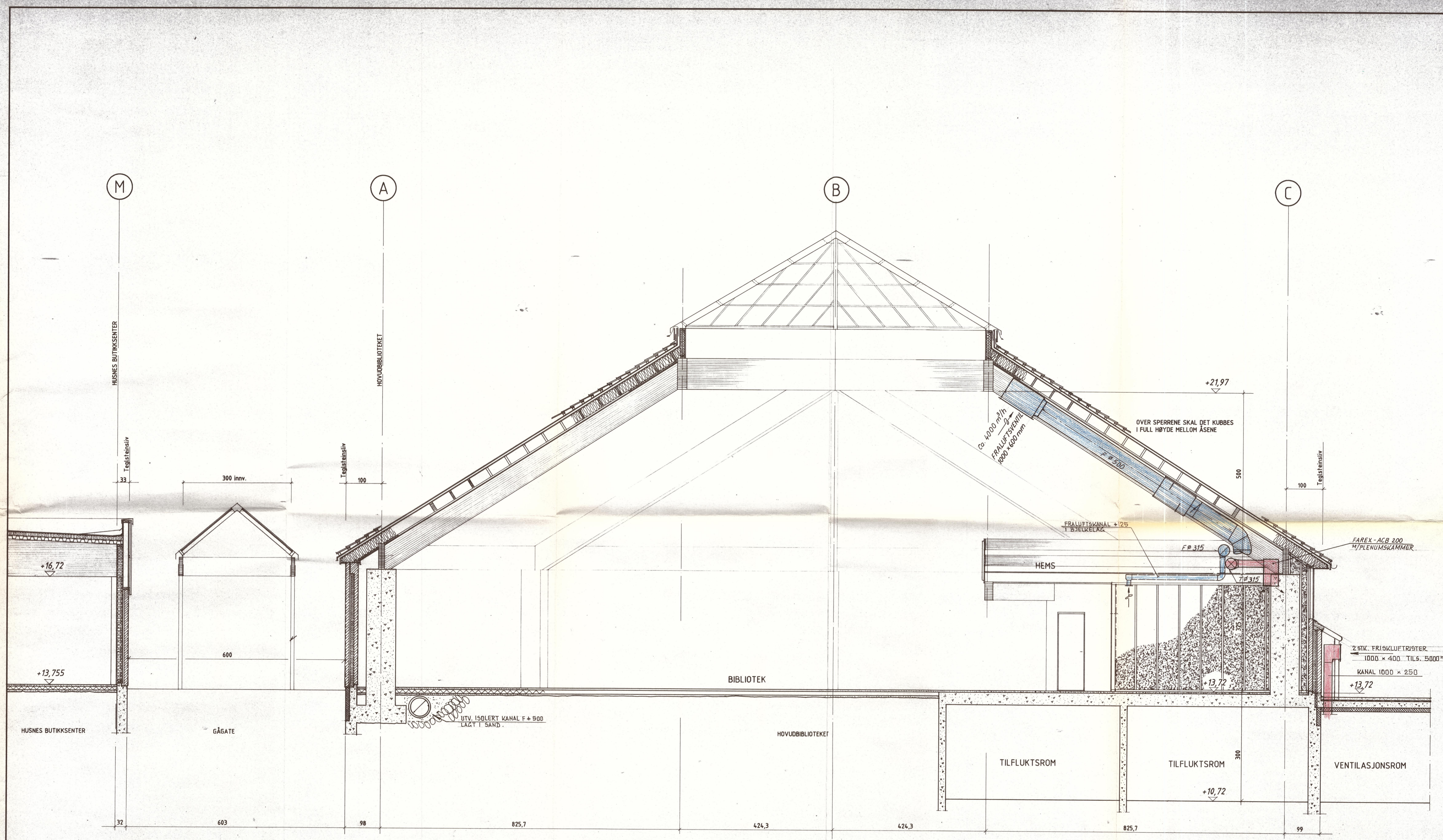
SNITT I AKSE 2
