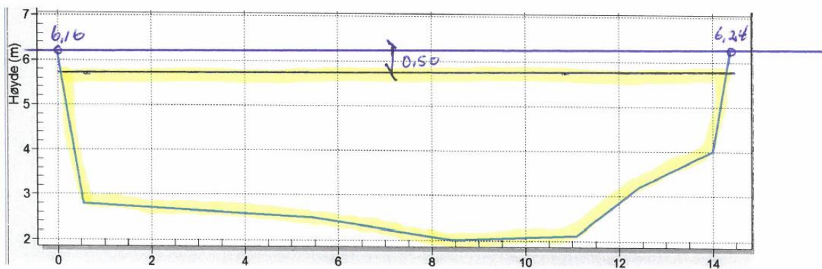
Dønnsaug bru (8)
