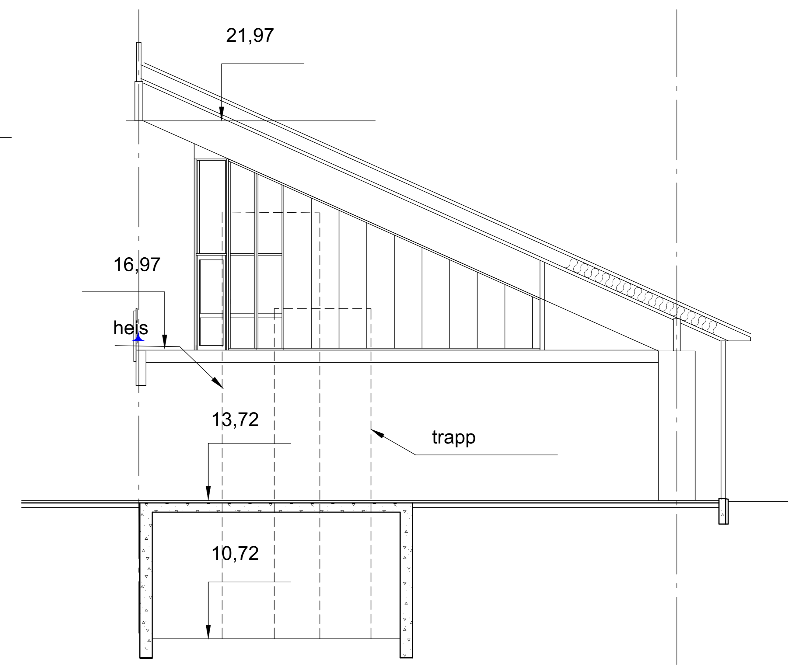
SNITT A-A
